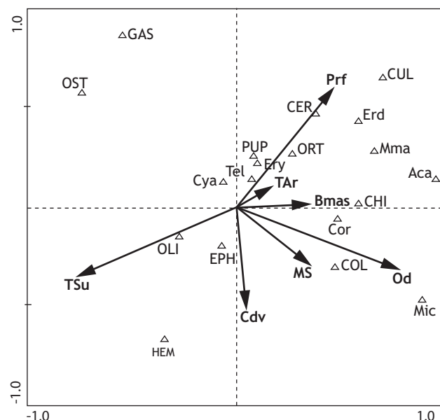
Figura 2 - Análise de correspondência canônica (ACC) envolvendo os macroinvertebrados amostrados junto à S. auriculata no Rio Guareí e os fatores ambientais, no período de março a dezembro de 2006. Legenda: Ceratopogonidae (CER), Chironomidae (CHI), Coleoptera (COL), Culicidae (CUL), Ephemeroptera (EPH), Gastropoda (GAS), Hemiptera (HEM), Oligochaeta (OLI), Orthoptera (ORT), Ostracoda (OST), Pupa de Diptera (PUP), Acanthagrion (Aca), Coryphaeschna (Cor), Cyanallagma (Cya), Erythemis (Ery), Erythrodiplax (Erd), M. marcella (Mma), Micrathyria (Mic), Telebasis (Tel), oxigênio dissolvido (Od), condutividade (Cdv), temperatura de superfície da água (TSu), temperatura do ar (TAr), profundidade (PRF), material em suspensão (MS) e biomassa (Bmas).
