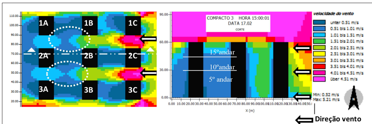
Figuras 15 e 16 - Seção horizontal no nível do 5º pavimento; Seção vertical – às 15h00 – Compacto 3. Fonte: Elaborada pelos autores.
