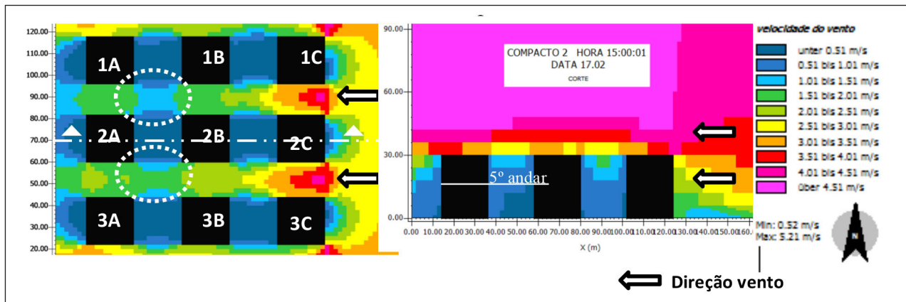
Figuras 11 e 12 - Seção horizontal no nível do 5º pavimento; Seção vertical – às 15h00 – Compacto 2. Fonte: Elaborada pelos autores.
