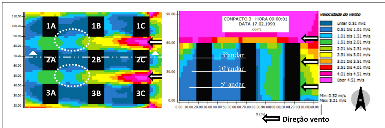
Figuras 13 e 14 - Seção horizontal no nível do 5º pavimento; Seção vertical – às 09h00 – Compacto 3. Fonte: Elaborada pelos autores.
